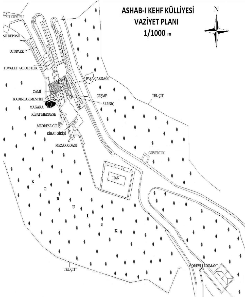
Şekil 1.1. Ashabü'l-Kehf Külliyesi Vaziyet Planı 194
