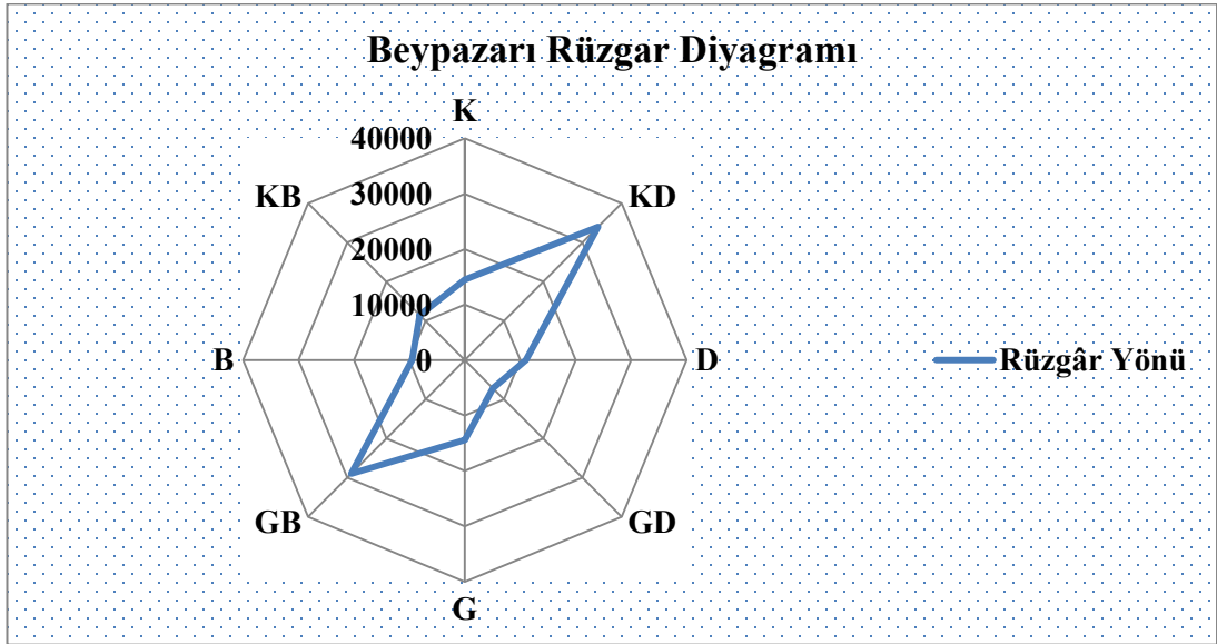
Şekil 36: Beypazarı meteoroloji istasyonu rzgr diyagramı
