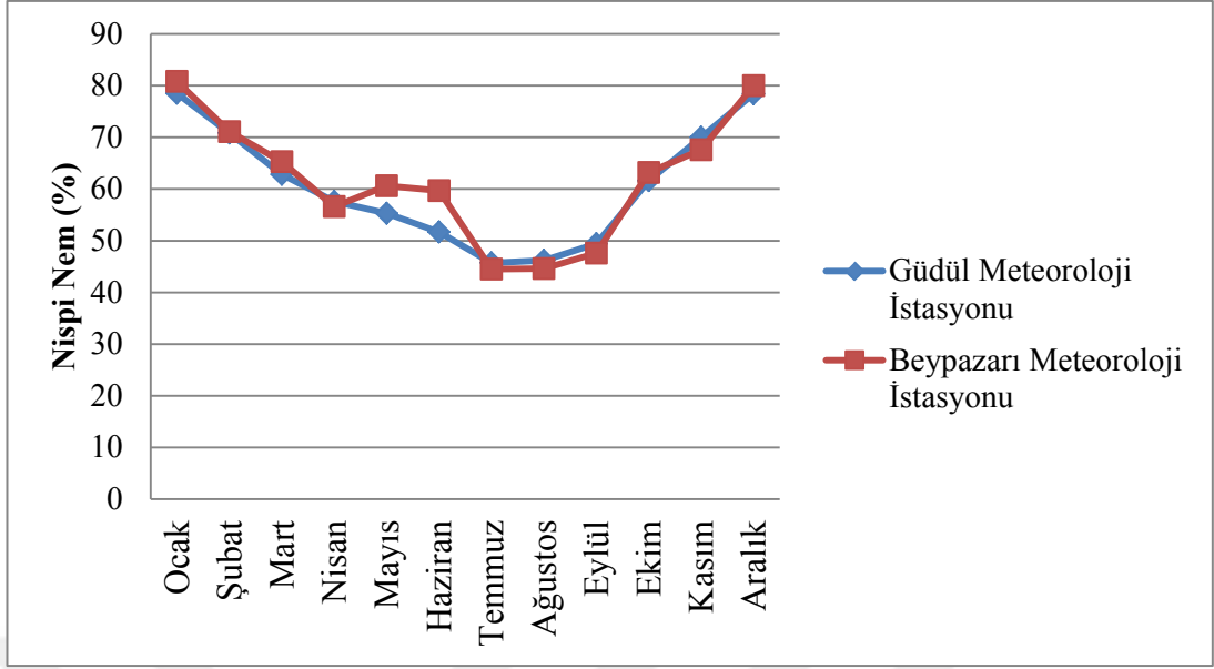
Şekil 35: Beypazarı ve Gdl meteoroloji istasyonu aylara gre ortalama nispi (baėlı) nem grafiėi
