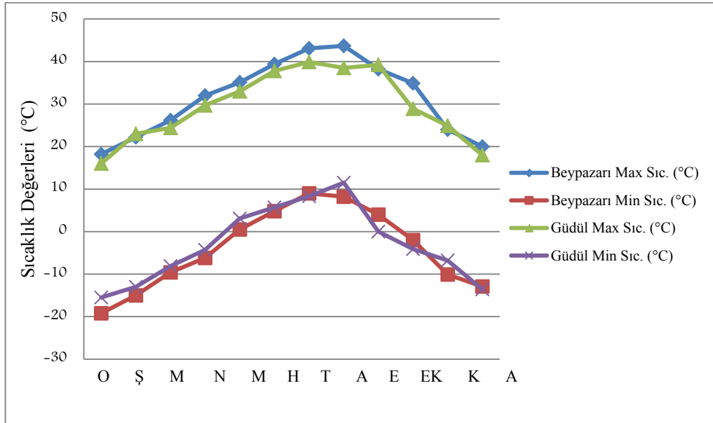
Şekil 30: Beypazarı ve Güdül meteoroloji istasyonları ortalama yüksek ve düşük sıcaklık grafiği
