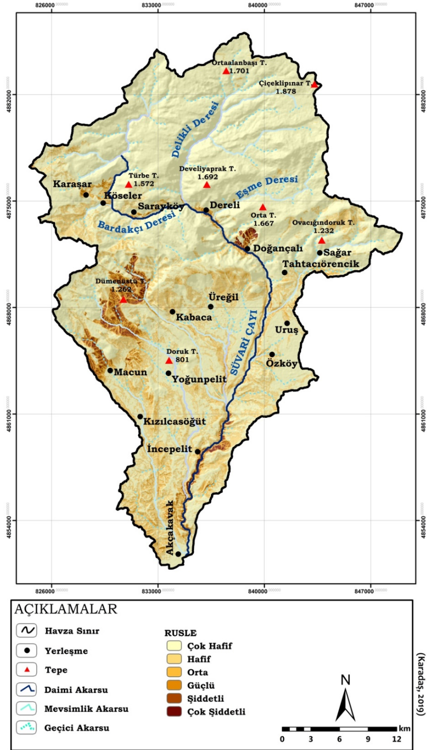
Şekil 86: RUSLE modeli erozyon duyarlılık haritası
