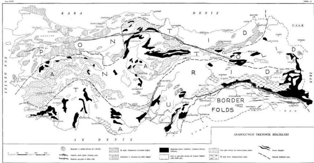
Şekil 8: Türkiye'nin kesitleştirilmiş tektonik haritası (Ketin, 1966)
