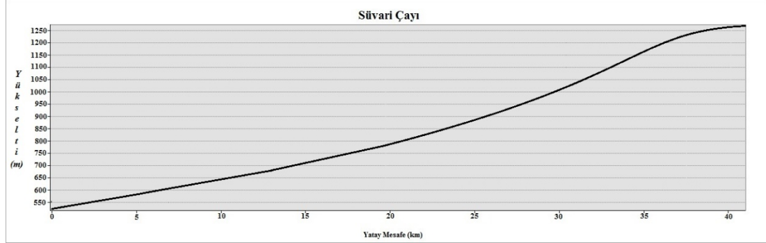
Şekil 72: Süvari çayı boyunca profili
